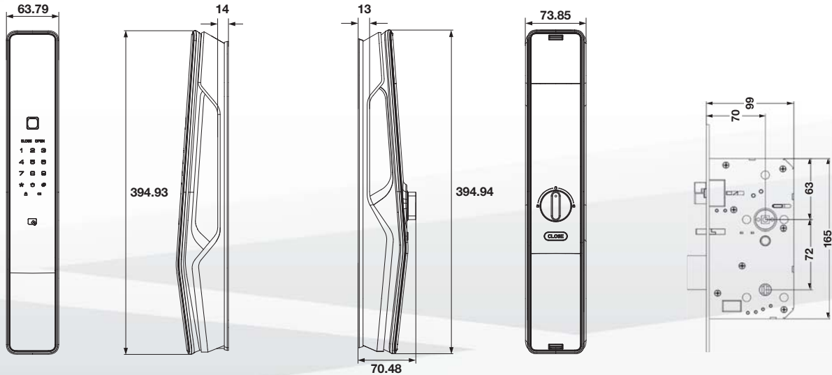
External Module โมดูลด้านนอกห้อง
